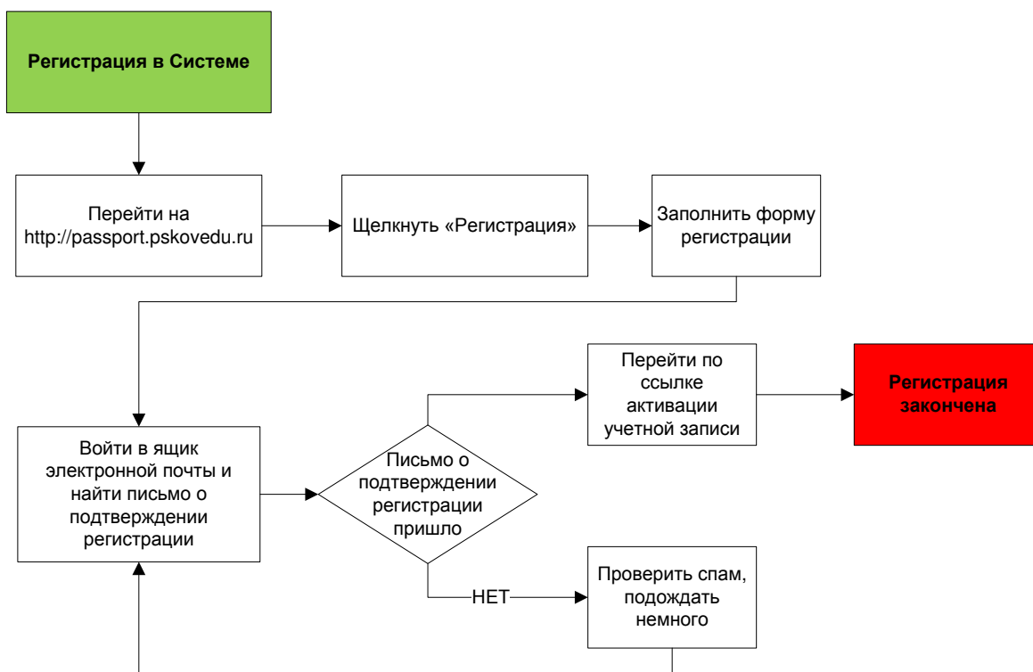
Рисунок 1 - Схема регистрации в Системе
